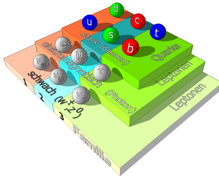
Abbildung 2: Das Standardmodell der Teilchenphysik
