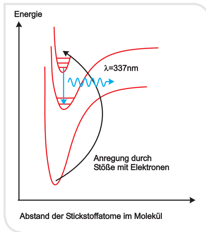
Abbildung 3: Molekülpotential eines Stickstoffmoleküls
